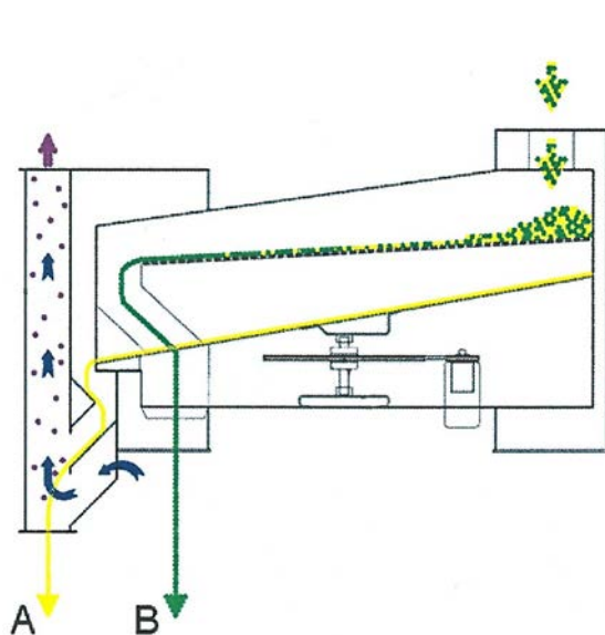
Typ SMA 202
