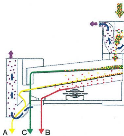
Typ SMA 203-3
