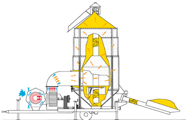
sušárna s přímým ohřevem
