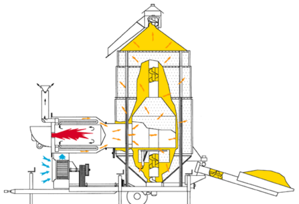
sušárna s nepřímým ohřevem
